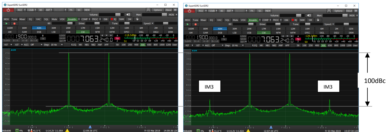
Bild 11: Zweitton-Signal mit 2x-20dBm am Eingang des Receivers, mit Dith & Rand (links) und ohne (rechts). Mit Dith & Rand beträgt die verzerrungsfreie Dynamik 100dBc, die IMD3-Signale verschwinden im Rauschen.
